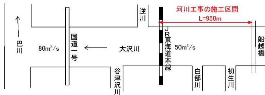
計画流量配分図
