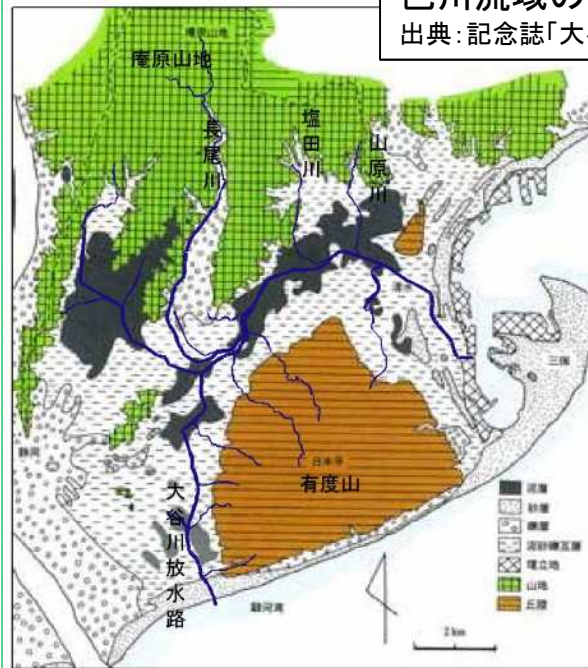
巴川流域の表層地質図
